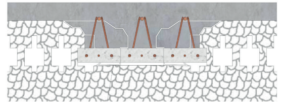
Les alvéoles permettent de jumeler, voire de tripler les poutrelles en gardant la sous-face décor.
